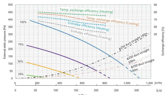
DIAGRAM LGH-80RVX3-E
