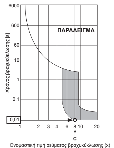
Σχεδιάγραμμα παραδείγματος
