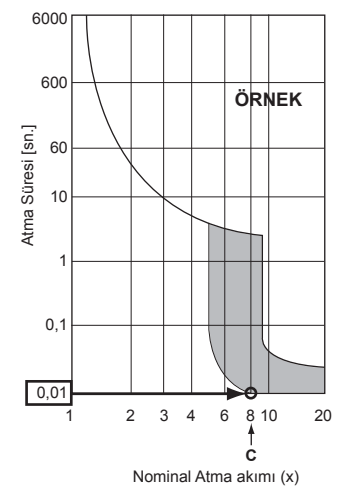
Örnek şema
